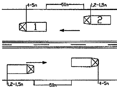
LOẠI 4 LÀN, 2 MÁI (MỖI BÊN 2 LÀN)
