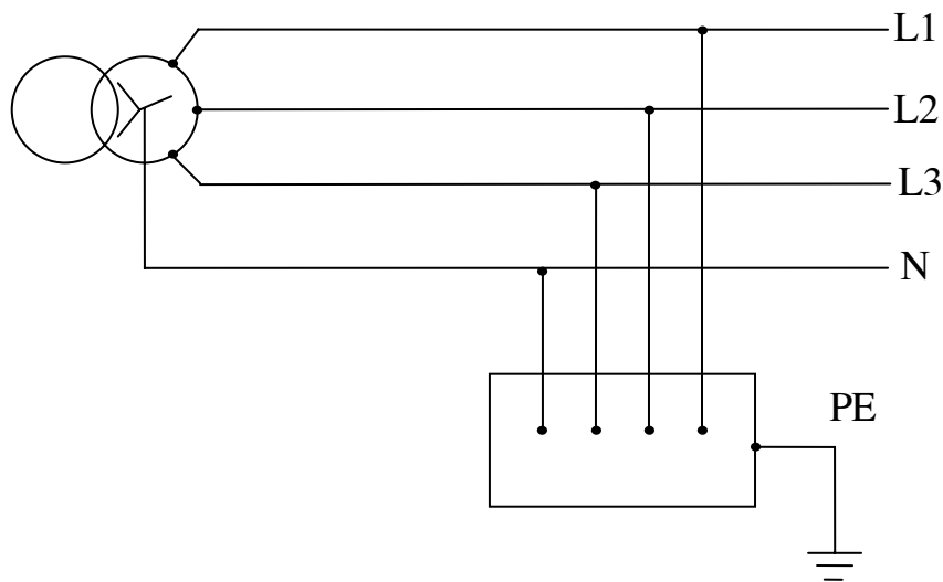
Hình 3.1B: Sơ đồ IT có dây trung tính .
