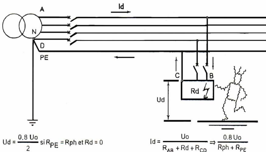
Hình 3C1 Dòng điện sự cố I_d và điện áp tiếp xúc U_d trong sơ đồ TN
